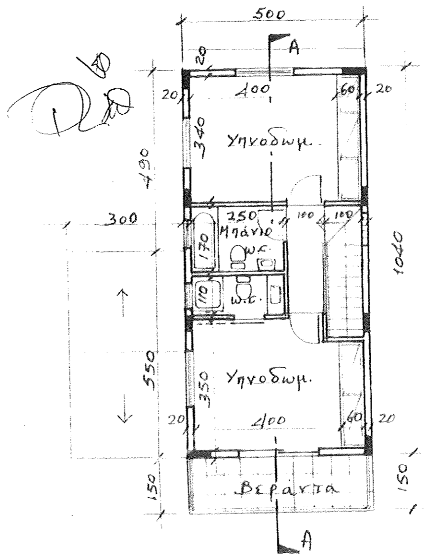
ΚΑΤΟΨΗ ΟΡΟΦΟΥ
