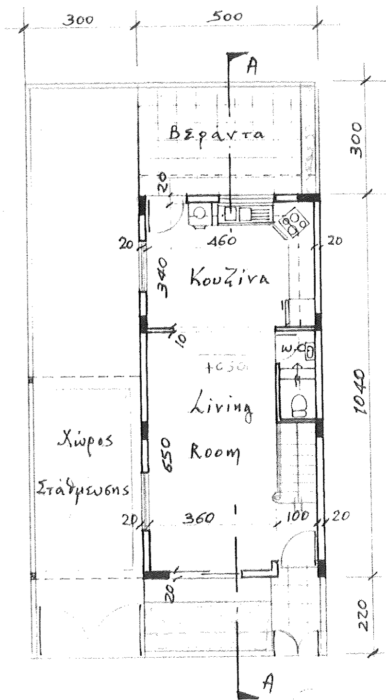
ΚΑΤΟΨΗ ΙΣΟΓΕΙΟΥ
