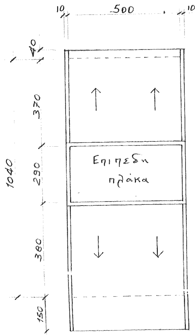
ΚΑΤΟΨΗ ΣΤΕΓΗΣ
